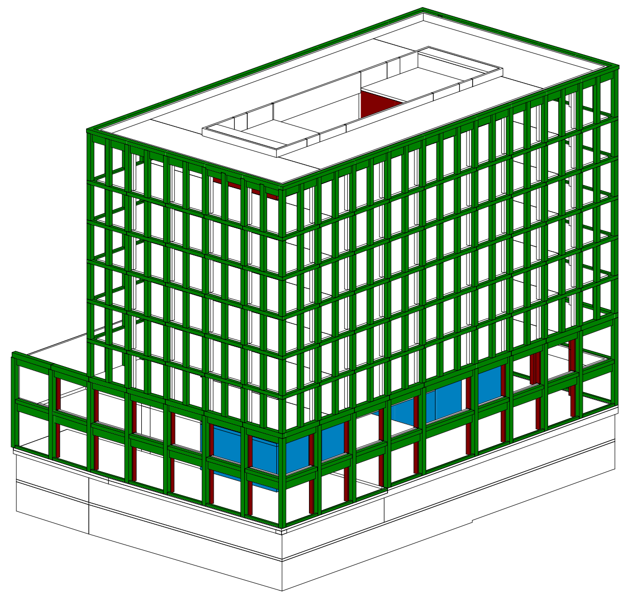
2 Bâtiment C - Vue 3D orientation SE
