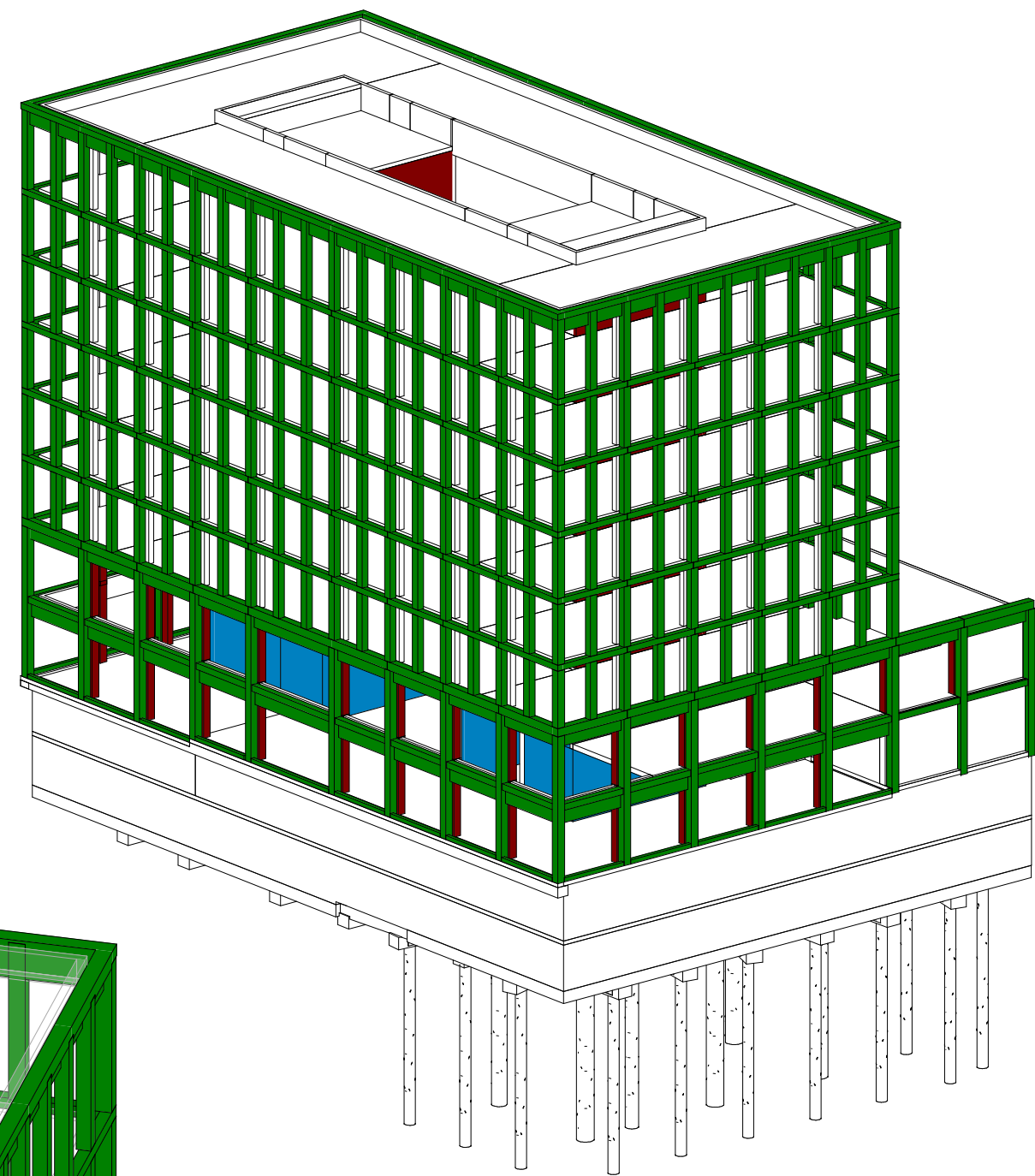
3 Bâtiment C - Vue 3D orientation NE
